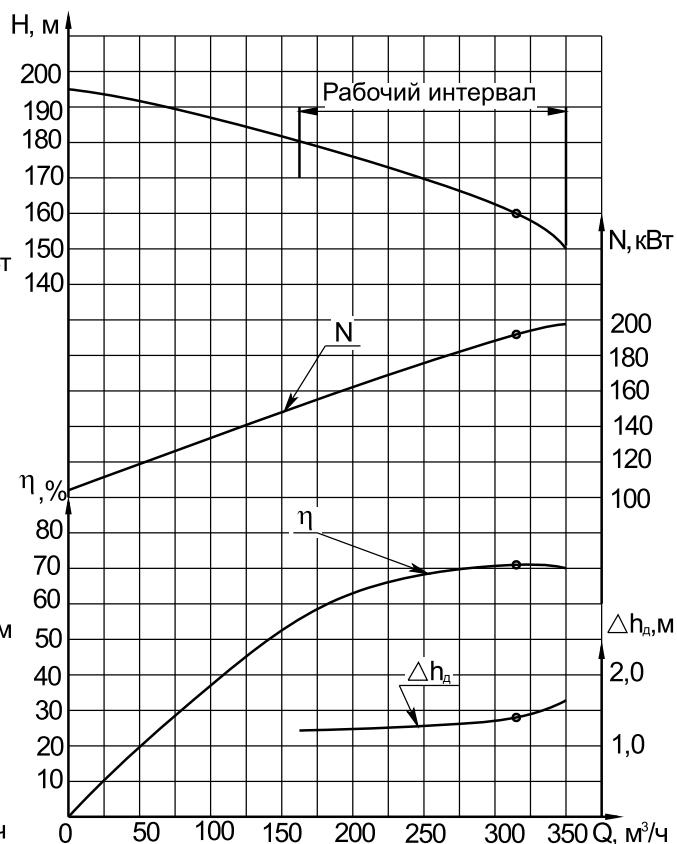
ХАРАКТЕРИСТИКА АГРЕГАТОВ 1КсВ 315-160-1
