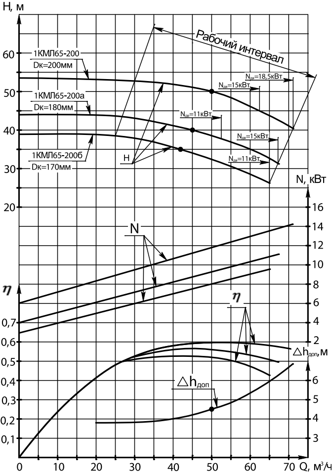
Характеристика насоса 1КМЛ65-200 на воде t=293K (20°C), ρ=1000кг/м³, n=48,3 с -1 (2900 об/мин)
