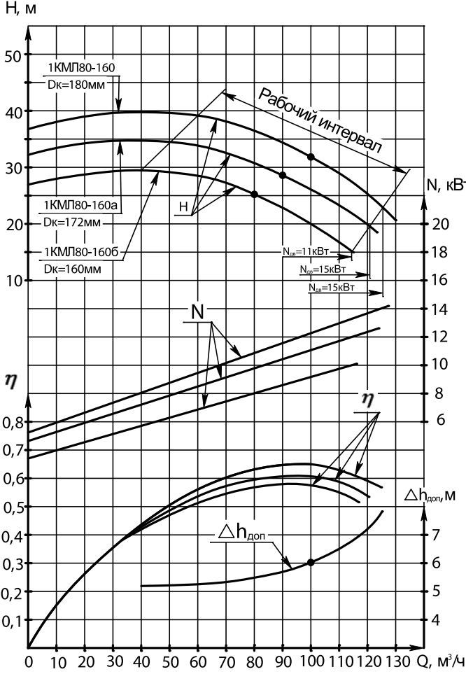
Характеристика электронасоса 1КМЛ80-160 на воде t=293K (20°C), ρ=1000кг/м³, n=48,3 с -1 (2900 об/мин)
